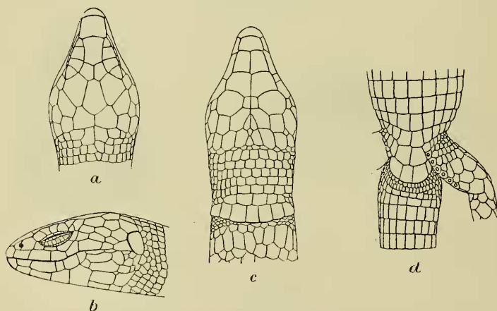
Proctoporus bogotensis .
